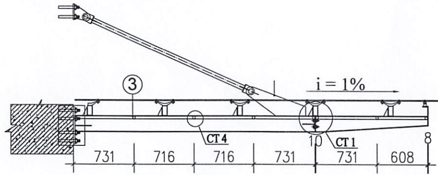
MẶT CẮT 1-1
