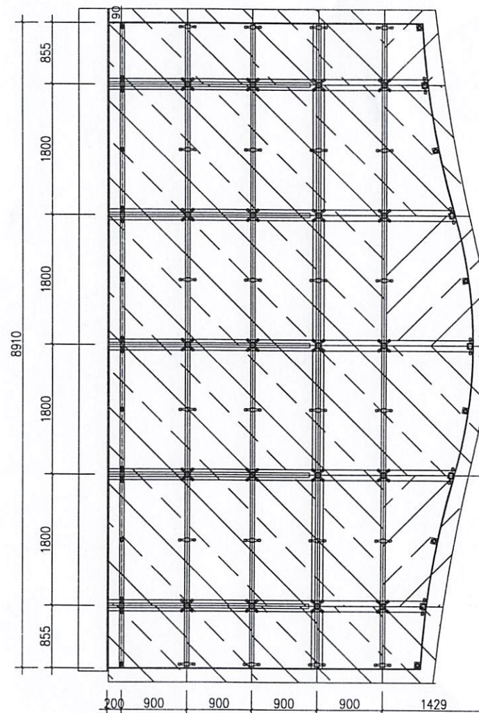
MẶT BẰNG MÁI KÍNH HIỆN HỮU
