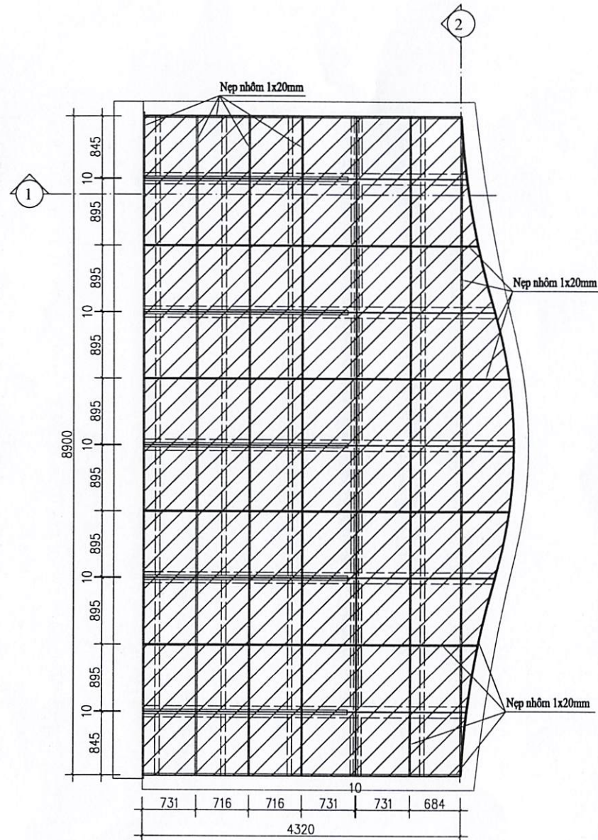
MẶT BẰNG ỐP TẤM ALUMINIUM DƯỚI KÍNH
