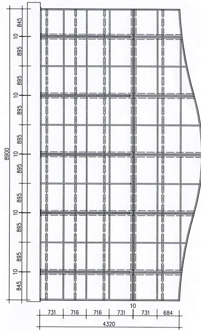
MẶT BẰNG KHUNG XƯƠNG ỐP TẤM ALUMINIUM
