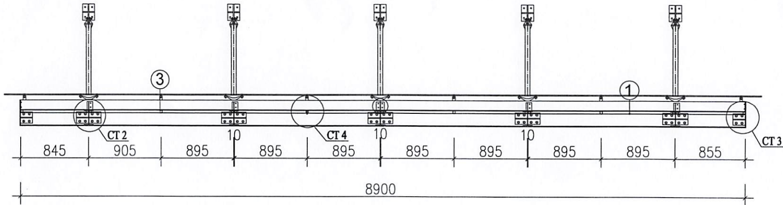
MẶT CẮT 2-2
