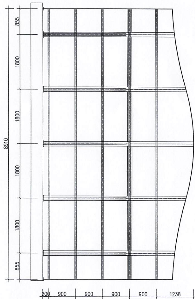
MẶT BẰNG KHUNG XƯƠNG MÁI KÍNH HIỆN HỮU
